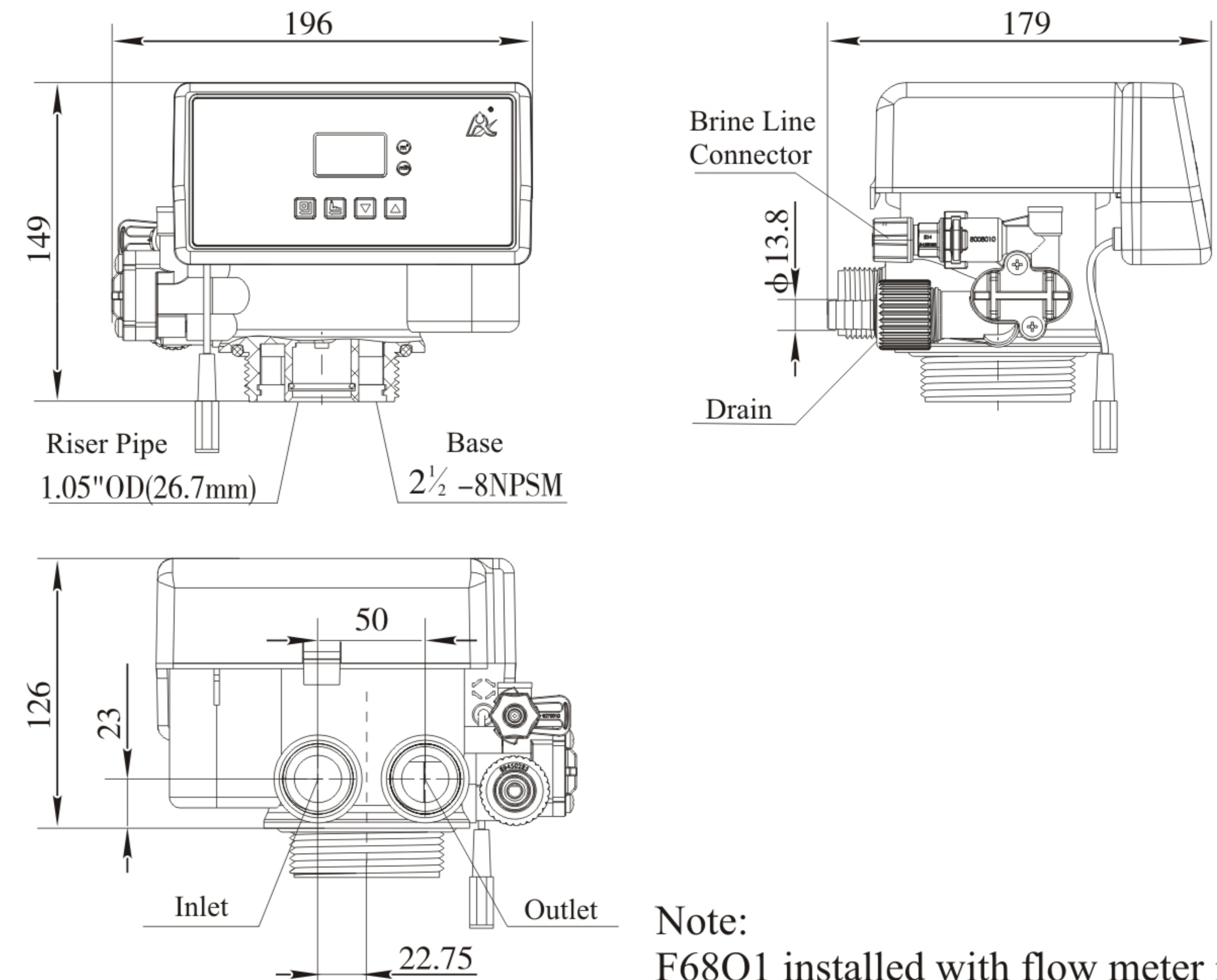
F68Q1 structure chart:
