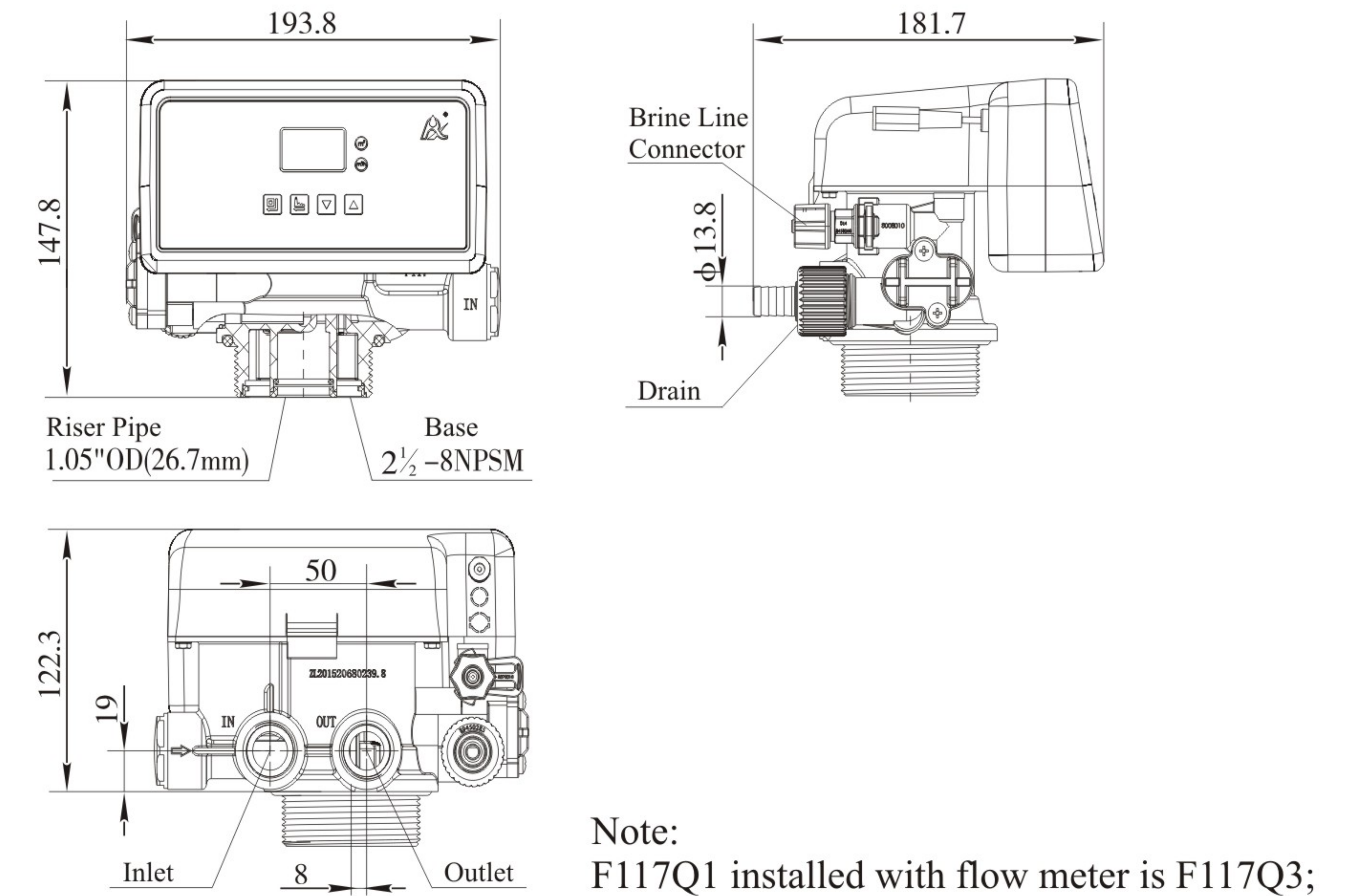
F117Q1 structure chart:
